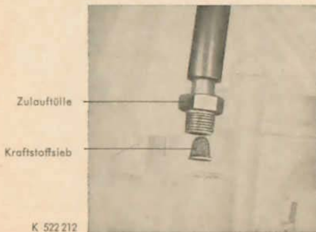
Abb. 12 Vergaserzulaufdüse mit Kraftstoffsieb
