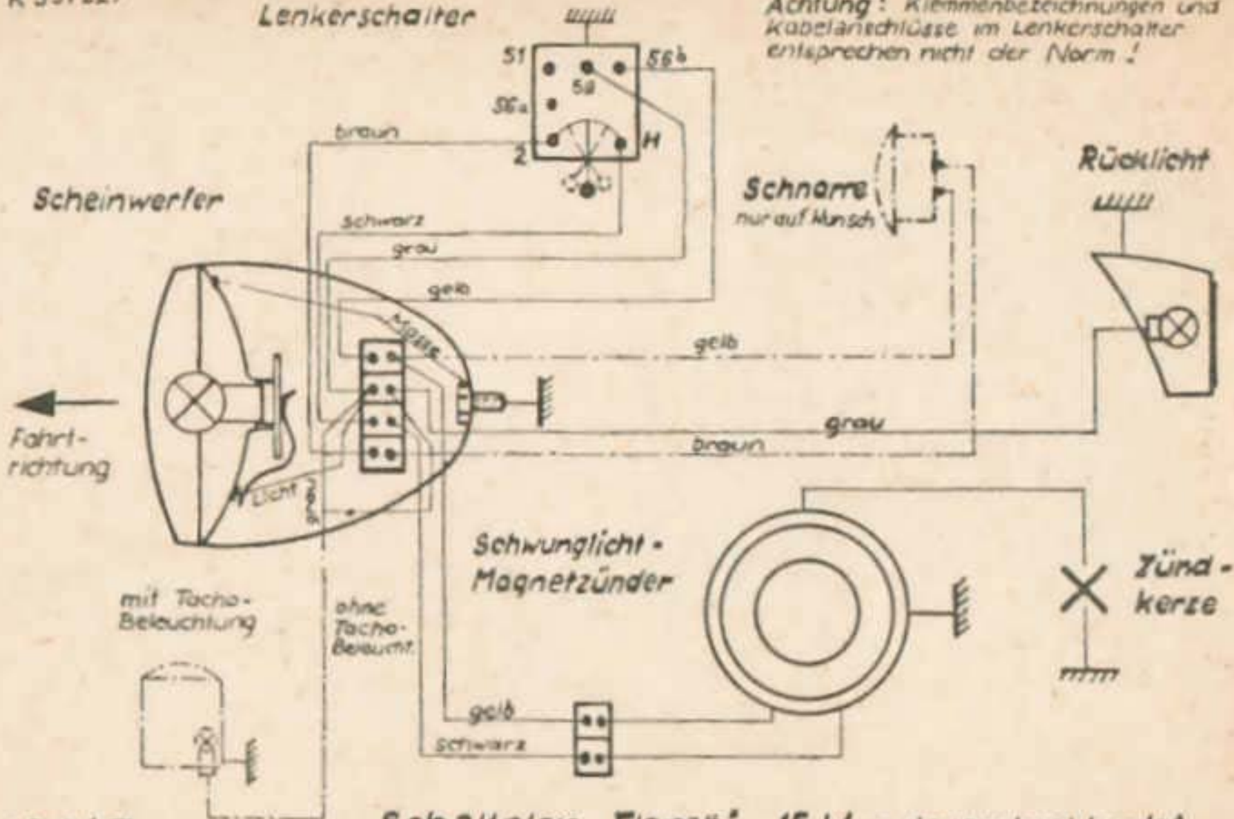
Abb. 27 Schaltbild für KREIDLER-Moped FLORETT
