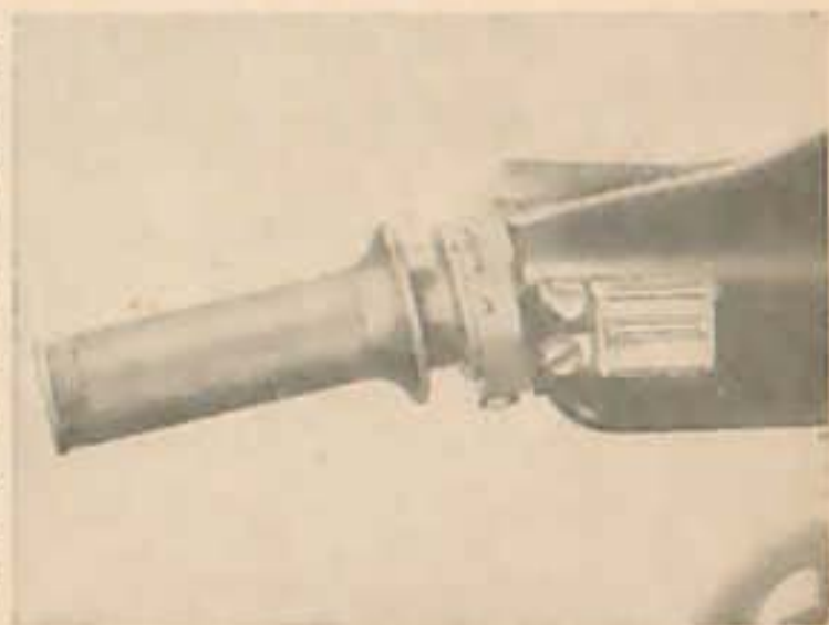
Abb. 5 Schaltdrehgriff in Leerlaufstellung
