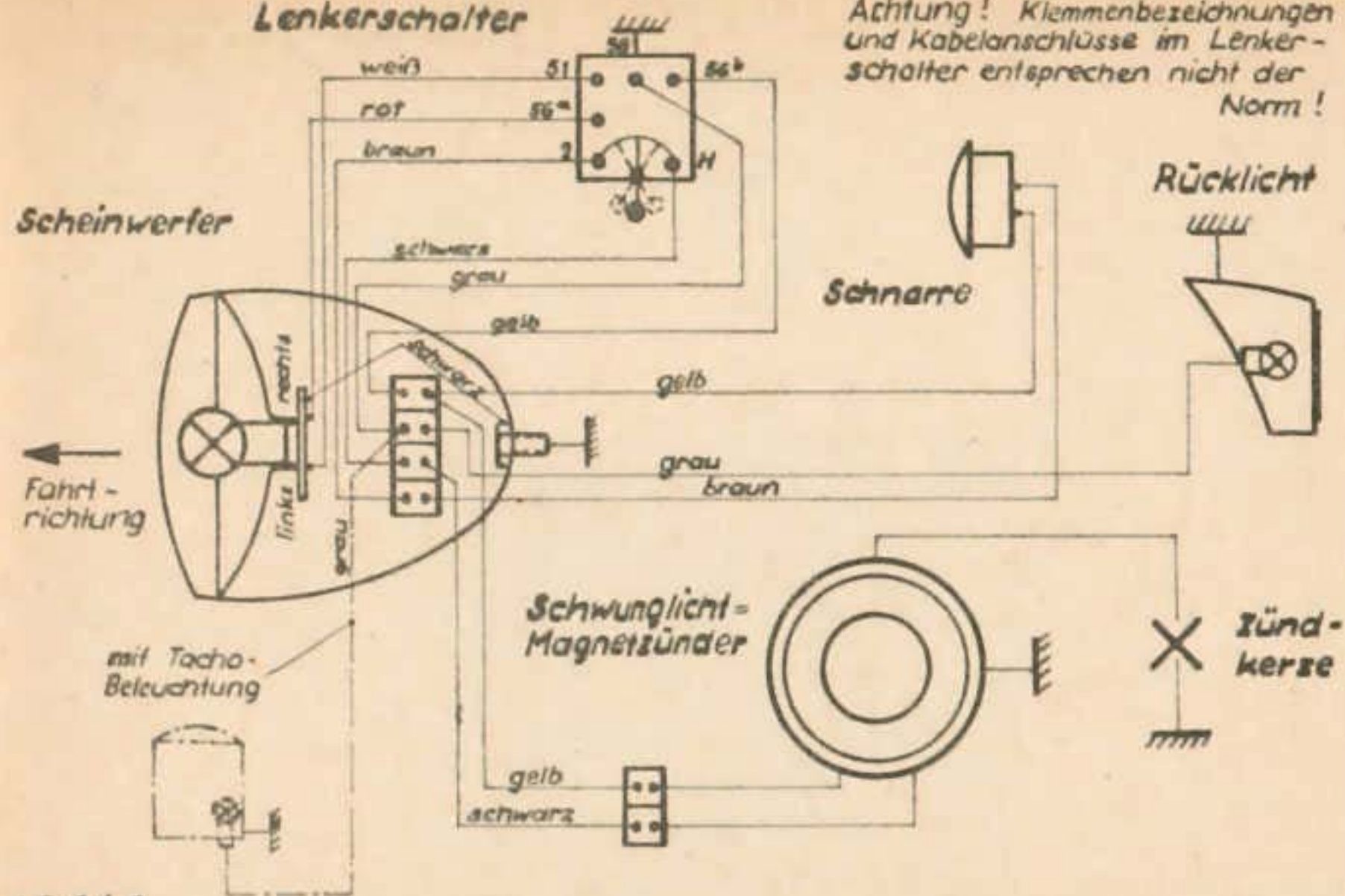
Abb. 27 Schaltplan für KREIDLER-Kleinkrafttrrad FLORETT
