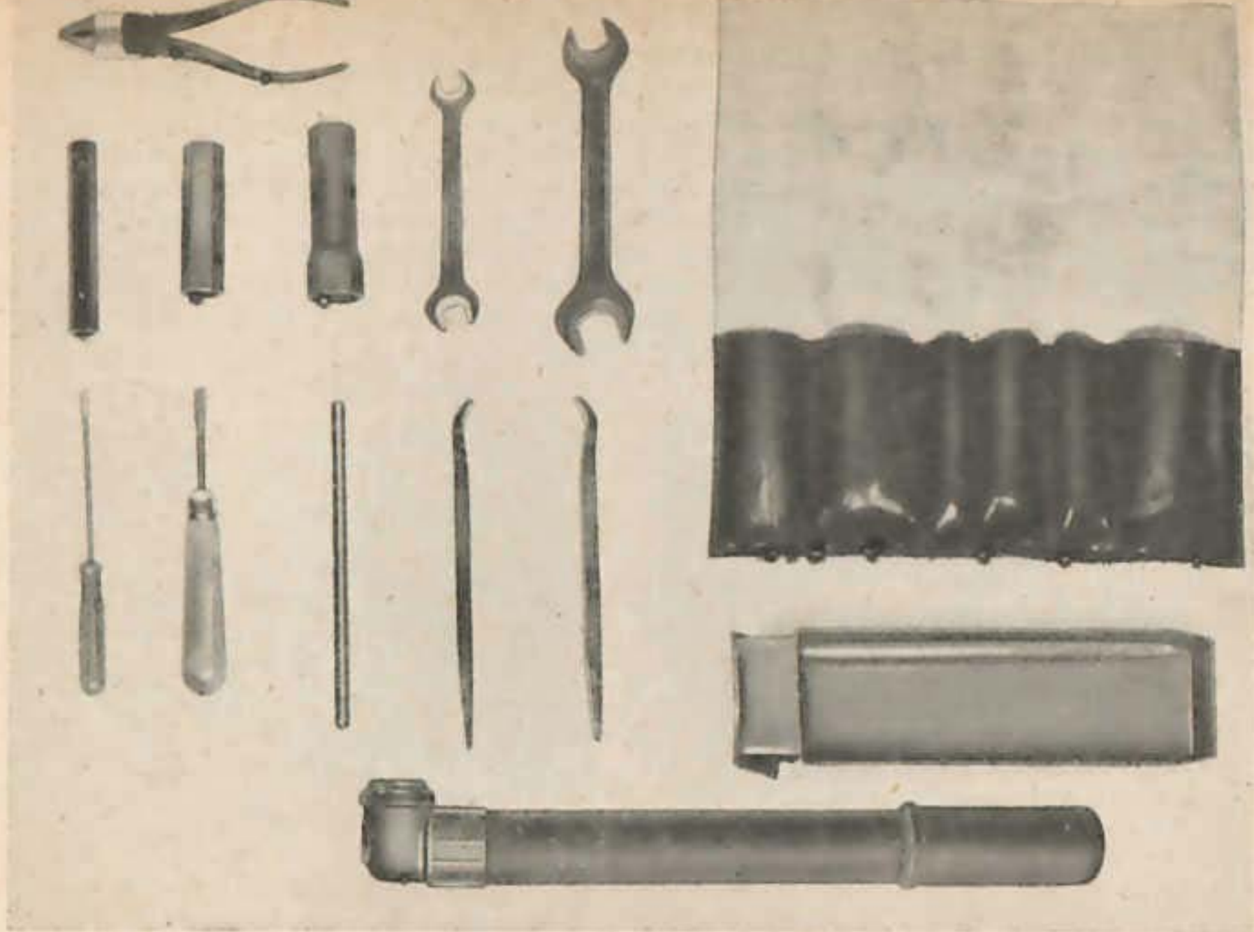
Abb. 34 Werkzeugsatz für Motorrad KREIDLER FLORETT
