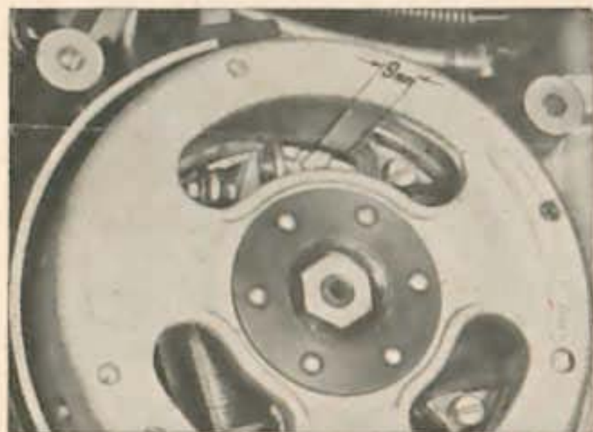
Abb. 15 Stellung des Polrades bei richtigem Polabrieb A
