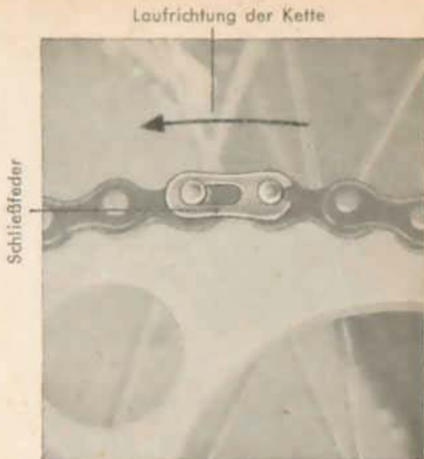
Abb. 41 Laufrichtung der Kette
