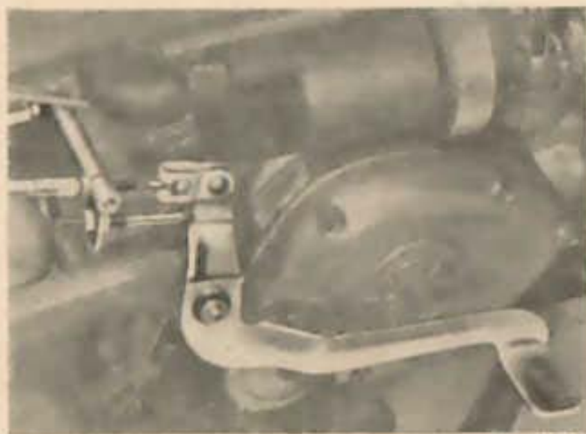
Abbildung 28 Nachstellen der Hinterradbremse
