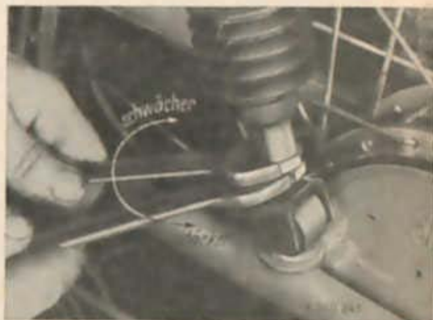
Abb. 46 Einstellen der Reibungsdämpfung
