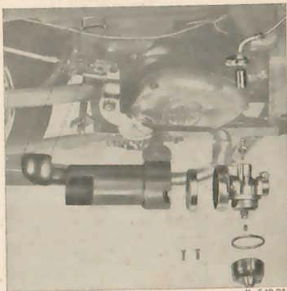
Abb. 11 Vergaser und Ansaugeräuschkämpfer (demontiert)
