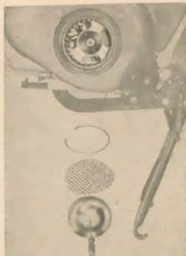
Abb. 14 Schwunglichtmagnetzünder (Gitter und Deckel abgenommen)
