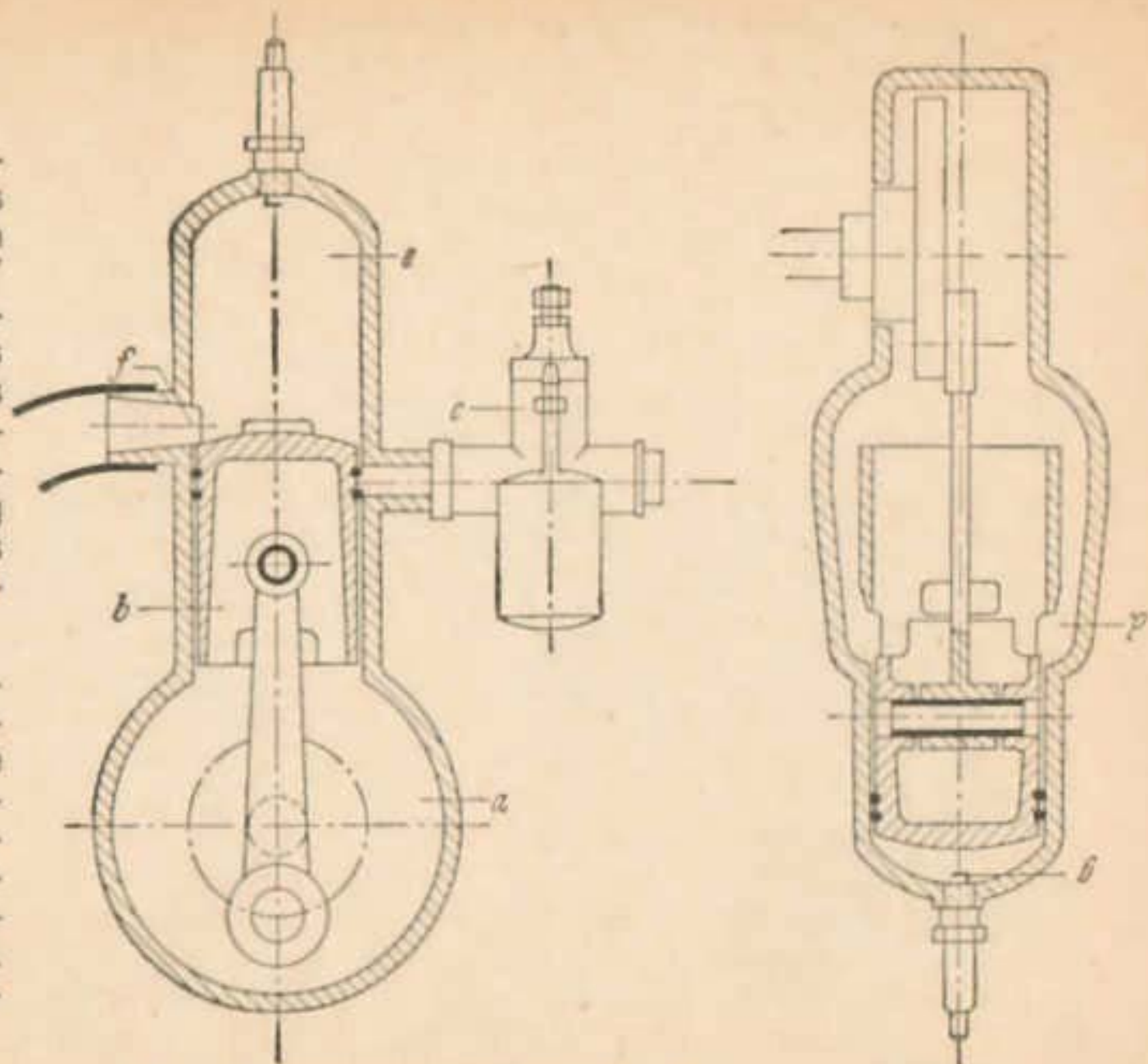
Abb. 8 Wirkungsweise des Zweitaktmotors
