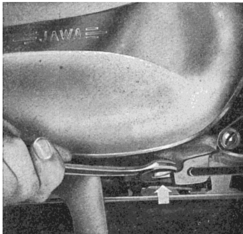
Obr. 10. Vypouštěcí šroub oleje z převodovky.
