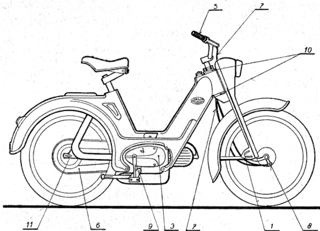
Obr. 9. Mazací plán - pravá strana.
