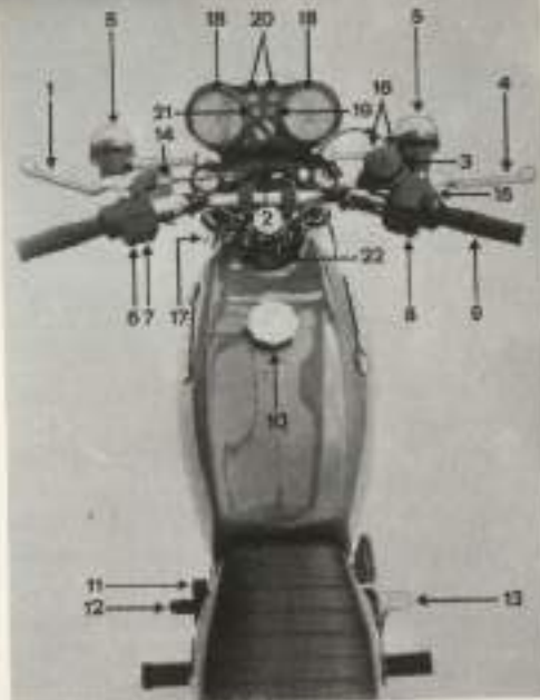
Fig. 1 - Disposizione comandi
