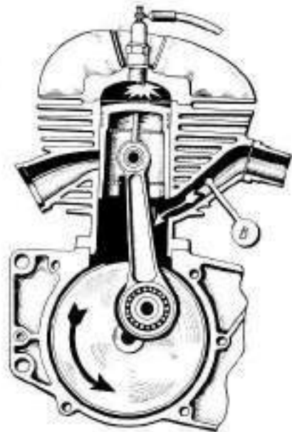
Рис. 30. Поршень движется в верхнем направлении
