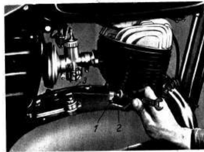
Рис. 46. Установление проволоки муфты сцепления
