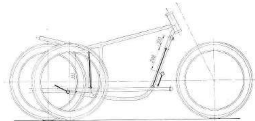
Рис. 63. Рисунок установки коляски мотоцикла в приблизительном направлении.
